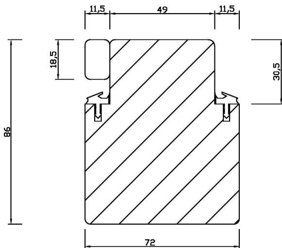
Oberlichtkämpfer
