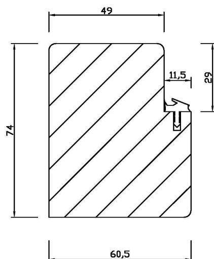
Sockelkämpfer
