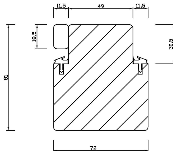
Aufrechte Kämpfer
