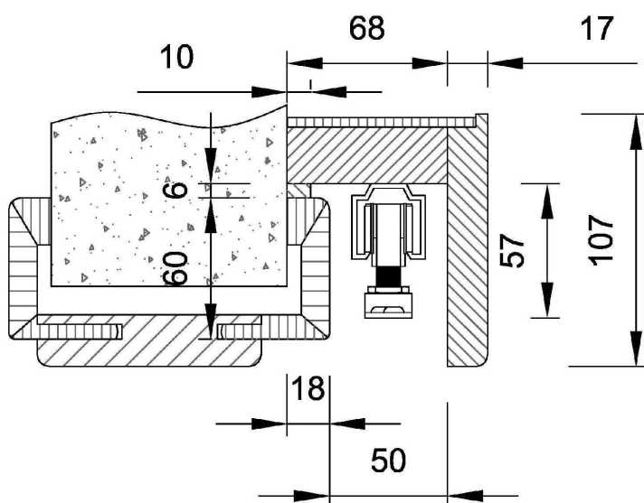
Laufkasten + Durchgangsfutter von Modell 20, bemaßt
