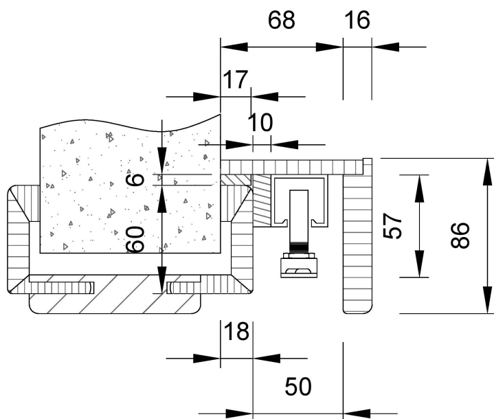
Laufkasten + Durchgangsfutter von Modell 20, bemaßt
