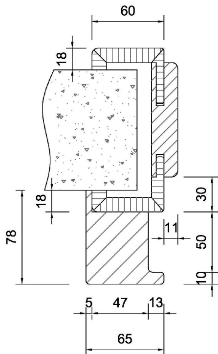
Anschlagkasten + Durchgangsfutter von Modell 20, bemaßt
