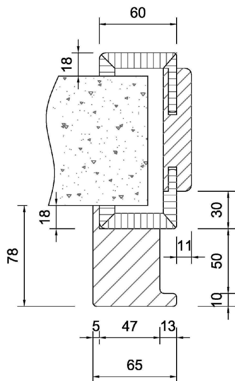
Anschlagkasten + Durchgangsfutter von Modell 20, bemaßt
