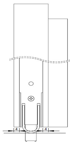
Bodendichtung Standflügel
