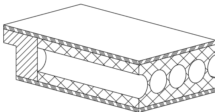
Röhrenspanplatte
